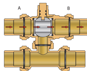
OPEN ACTUATOR
