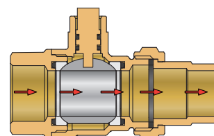
OPEN ACTUATOR
