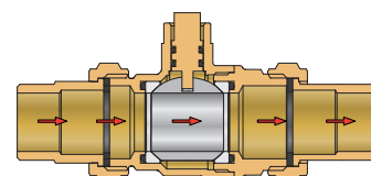
OPEN ACTUATOR
