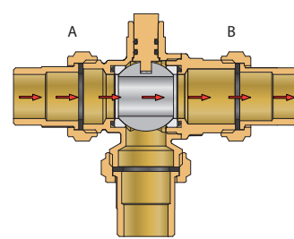
OPEN ACTUATOR
